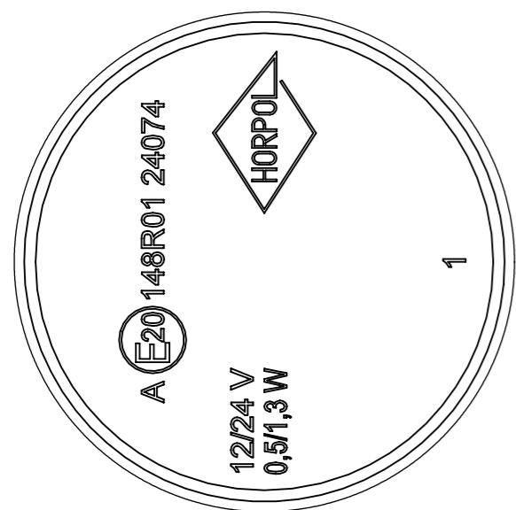
SZCZEGÓŁ A
