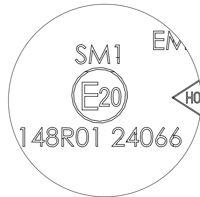
SZCZEGÓŁ A SKALA 4 : 1
