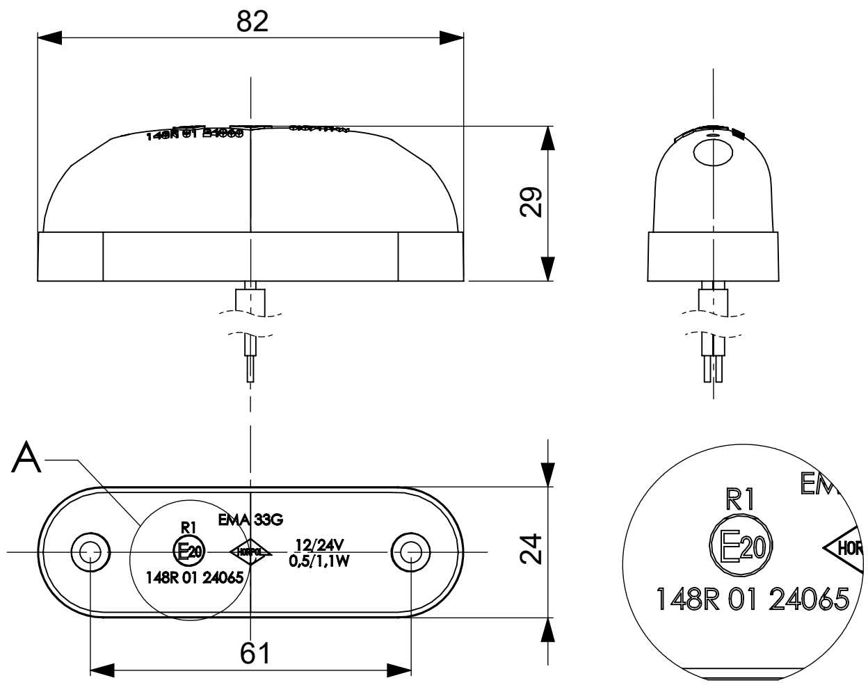
SZCZEGÓŁ A SKALA 2 : 1
